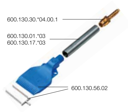
600.130.56.01 kiegészítővel *01 = 1.0711 / 17 = AISI 316Ti / 30 = réz
