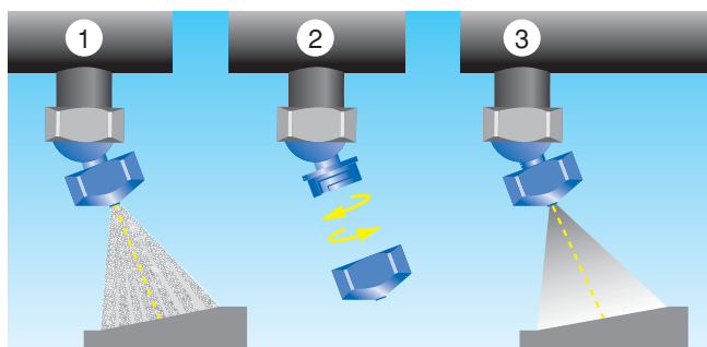
LECHLER MEMOSPRAY®: a fúvóka egy kézmozdulattal cserélhető - a szórásirány megmarad.
