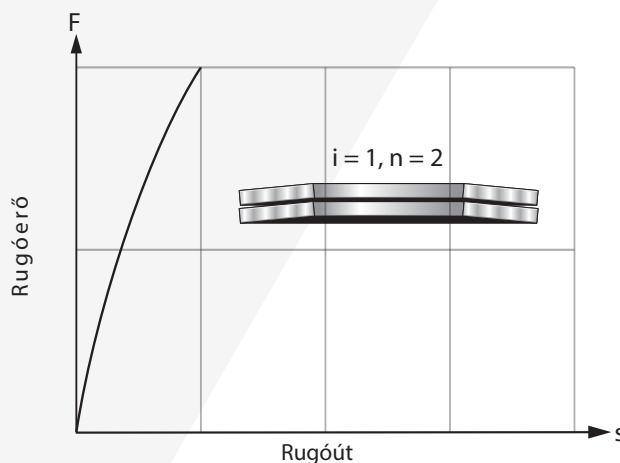
Tányérrugó-oszlop jelleggörbéje 2-szeres azonos irányú rétegezéssel. ▷ azonos út, 2-szeres erő.
