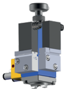
BS 25 SV Mini 15 automatic, flat grid / 2x pilot control valve
