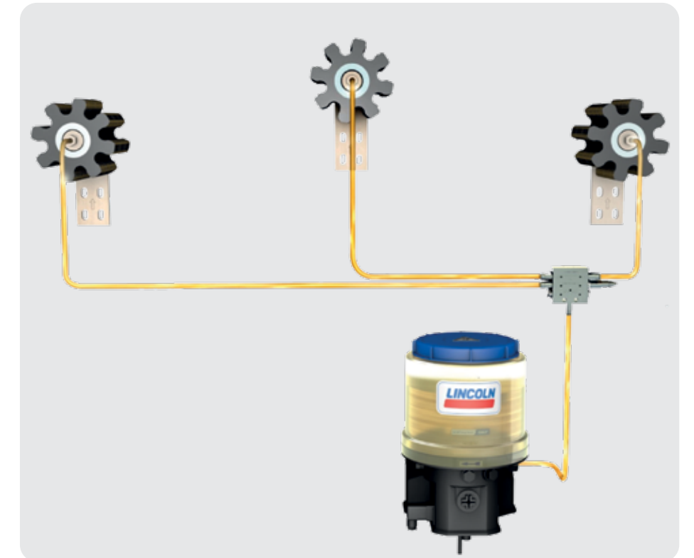
Daru fogaskoszorú automata kenése
