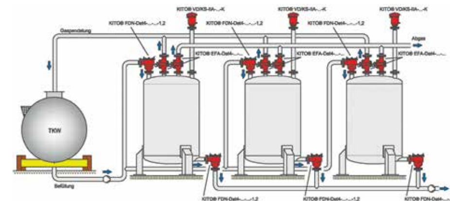
Tartálykocsi ürítő berendezés
