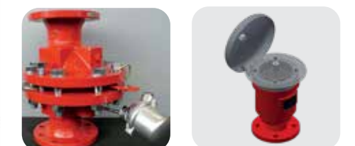
KITO biztonsági tartályarmatúrák
