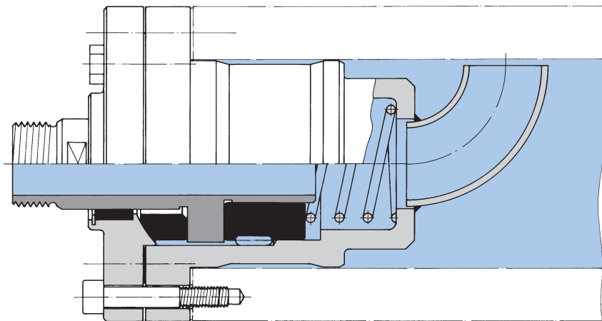
HW 125 K-24: integrált görgős csőcsap a visszaáramló hűtővízhez.
