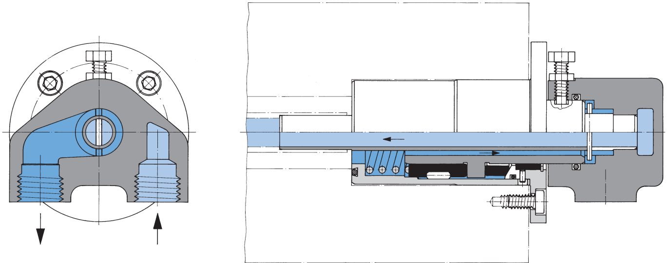
HW 225 K74: integrált görgős elosztó csőcsap a be és kimenő ághoz.
