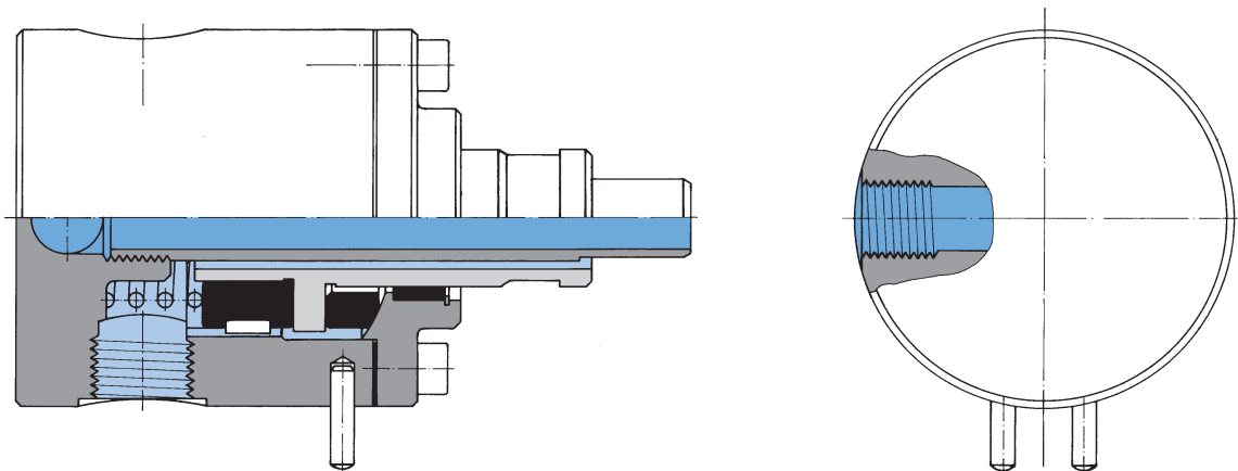
HW 225 K-27: Kompakt forgócsatlakozás duplacsatlakozással.
