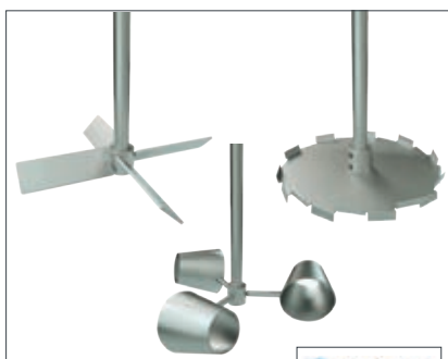
Keverőelemek
