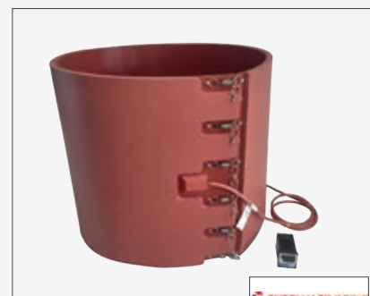
Fűtőpaplank, fűtőköpenyek
