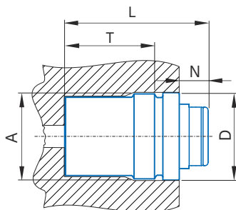
VN Verschlussnippel Self sealing adaptor
