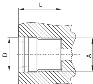
VK Verschlusskupplung Self sealing coupling
