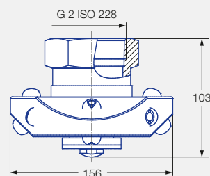
Innengewinde
