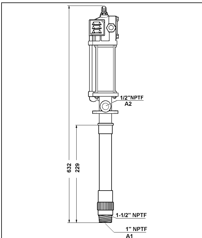
Pumpe Nr. 282396
