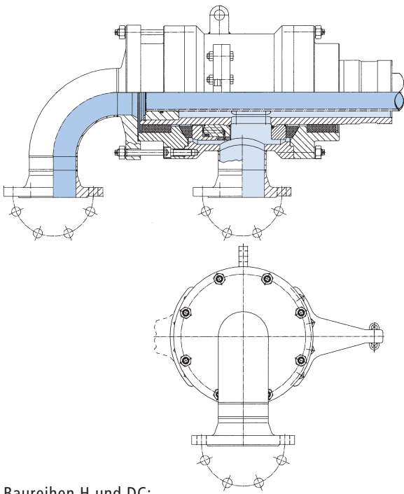
Baureihen H und DC: Geeignet für besonders große Dampfmenen. Lieferbar bis DN 350.
